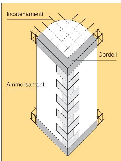
Nell'immagine: ammassamento della muratura in corrispondenza dell'angolo; realizzazione di cordoli in c.a. resistenti a trazione; incatenamenti al livello dei solai con estremità efficacemente ancorate ai cordoli.
